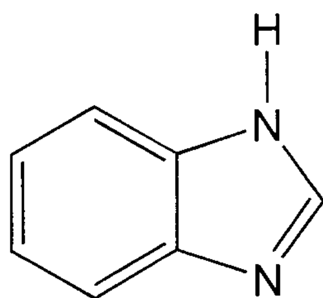
Benzimidazole
