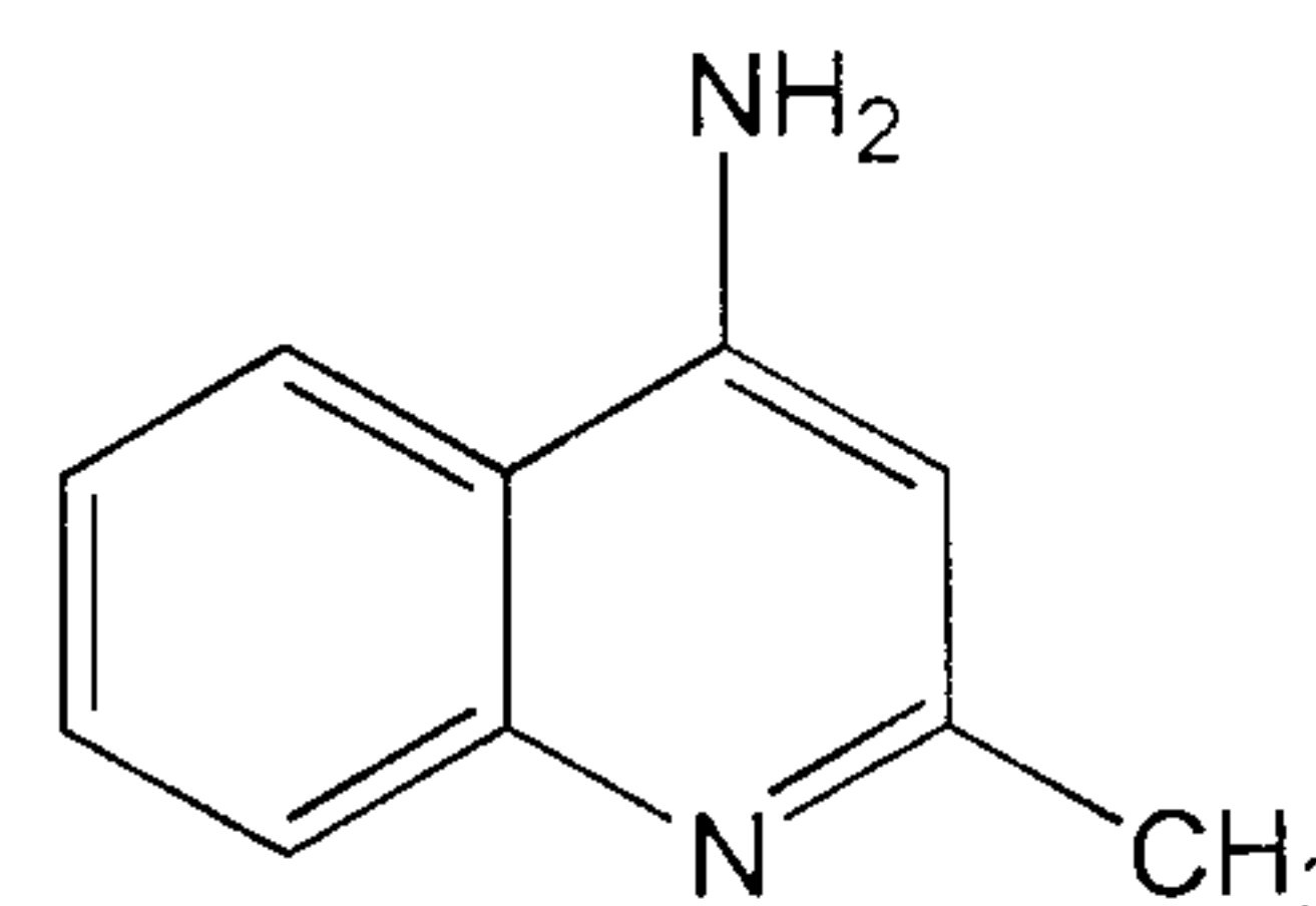
4-Amino quinaldine
