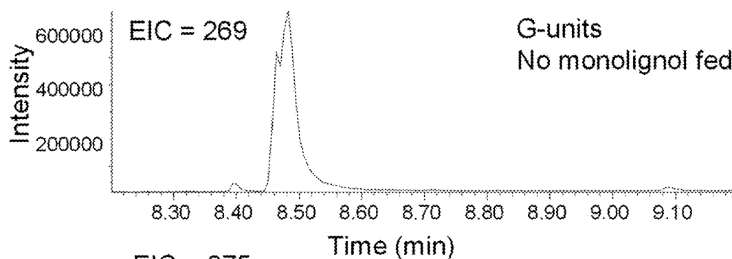
FIG. 6E m/z
