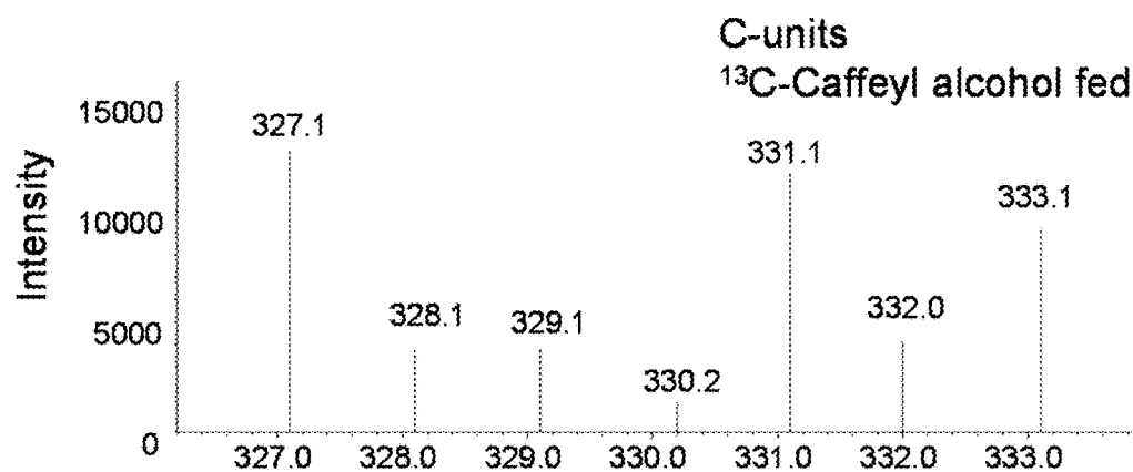
FIG. 6E m/z
