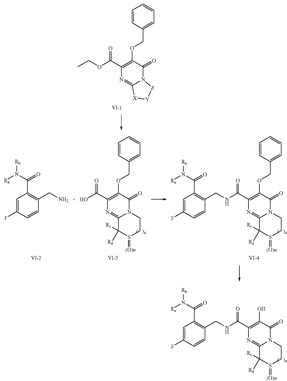
Scheme VI
