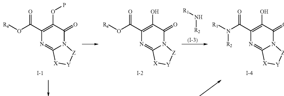
Scheme I.
