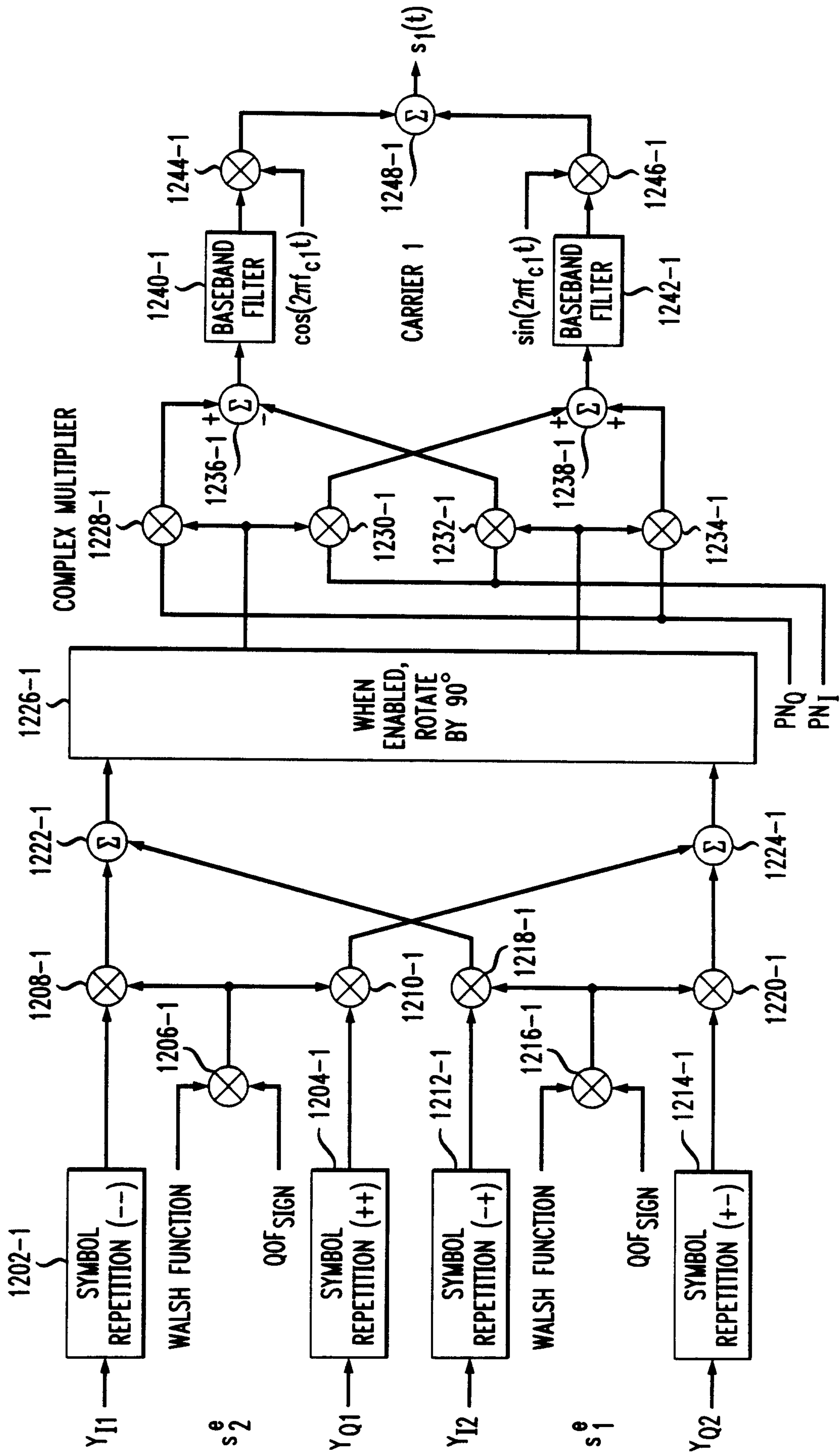
FIG. 12A P/O ANTENNA 2
