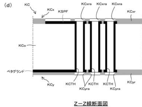
Z-Z線断面図
