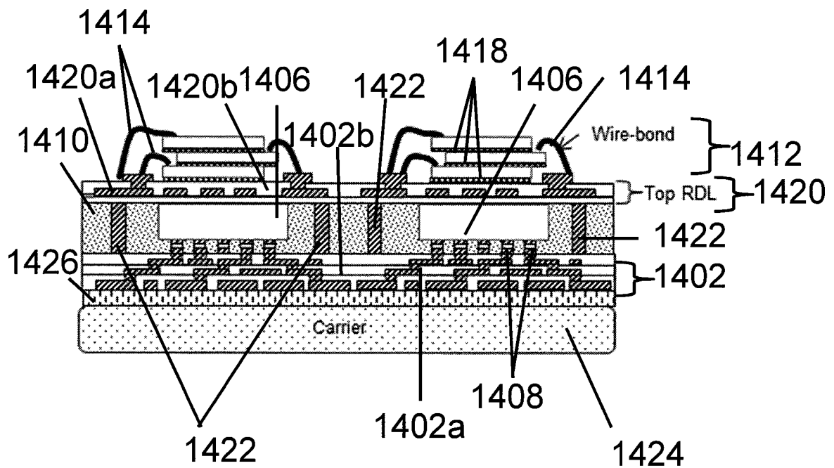
(g) Top RDL & UBM layer
