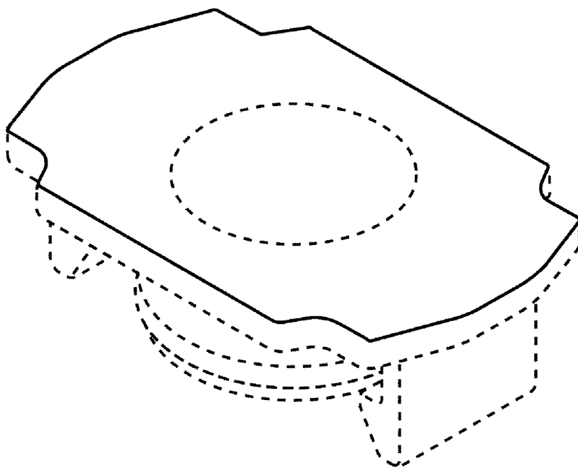
【立體圖】
