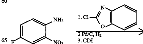
Scheme III:
