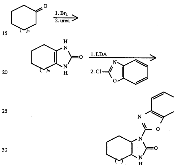
Scheme I:
