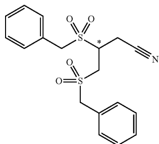
3,4-bis-benzylsulfonylbutanenitrile
