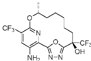
(composé 11) ,
