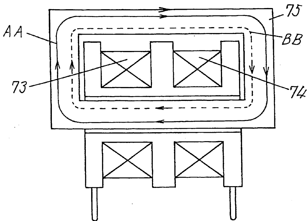
F i g . 3 2 P R I O R A R T
