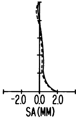
FIG. 4(a)
