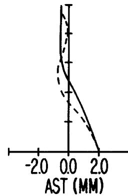
FIG. 4(e)
