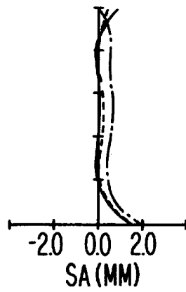
FIG. 2(d)
