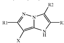
Imidazo[1,2-b]pyrazole
