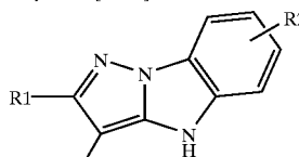
Pyrazolo[1,5-a]benzimidazole
