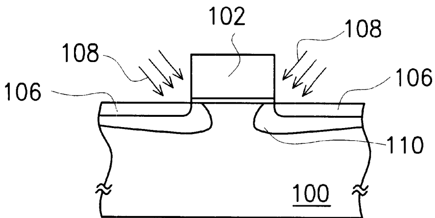
FIG. 1B(PRIOR ART)
