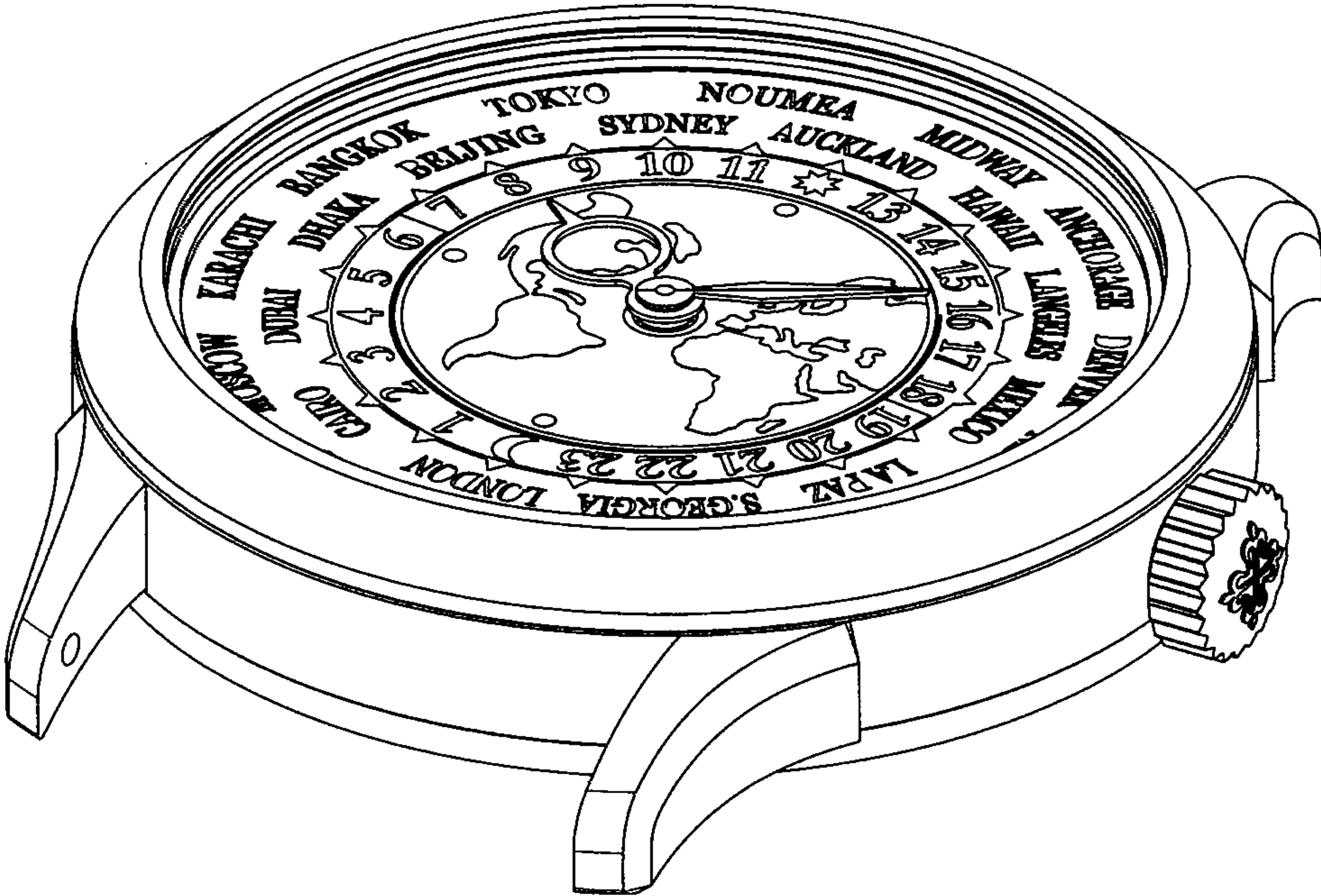
【立體圖】
