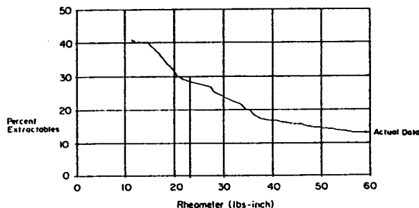
Rheometer vs. Percent Extractables Actual Determinations
