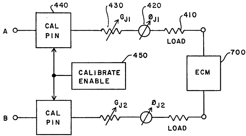
Fig. 4 ECM INTERFACE
