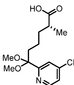
Verbindung 21.
