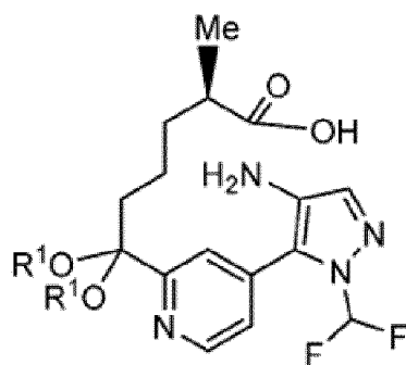
Composé 10 ;
