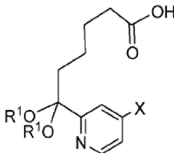
Composé 6
