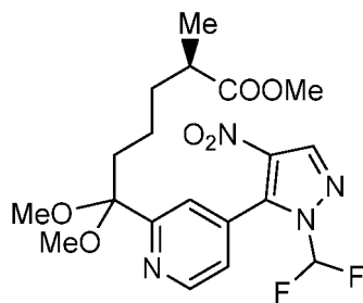
Verbindung 33.
