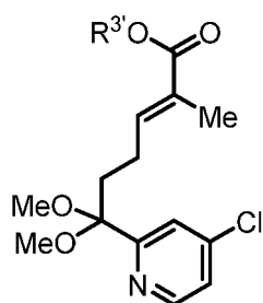
Composé 19
