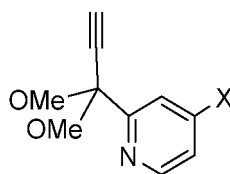
Verbindung 30
