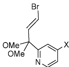
Verbindung 31
