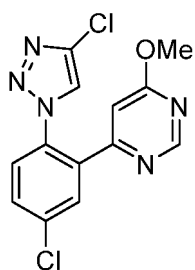
Composé 47 ;
