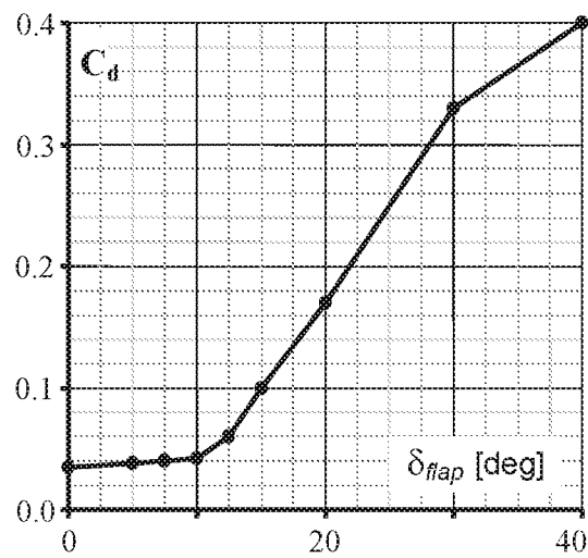
Fig. 17(b) airbrake drag
