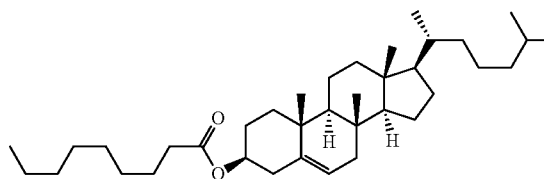
(Op-9)
