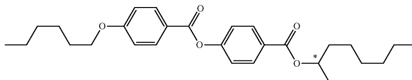
(Op-5)
