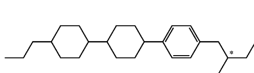
(Op-5)
