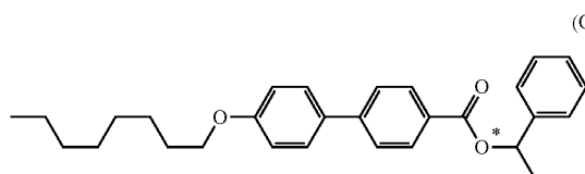
(Op-7)
