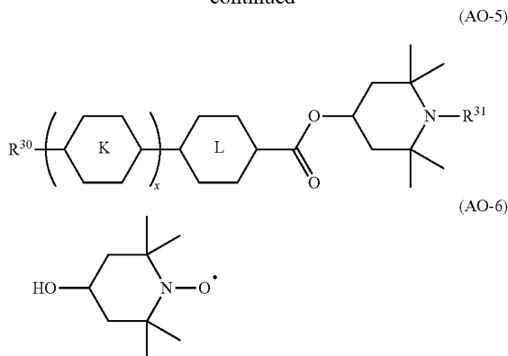
(AO-5)
