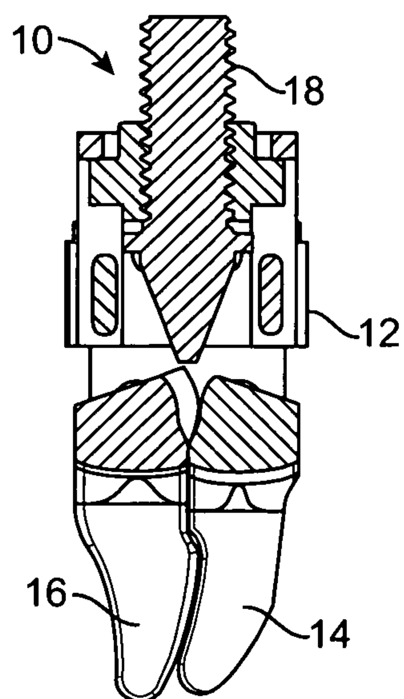
SECTION A-A
