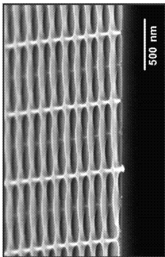
TiO 2 Grids
