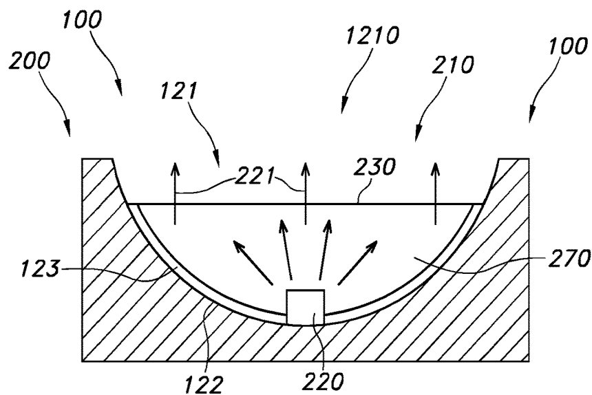
FIG. 2H
