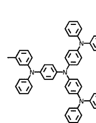
m-MTDATA
