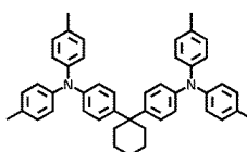
TAPC
