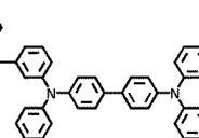
TPD
