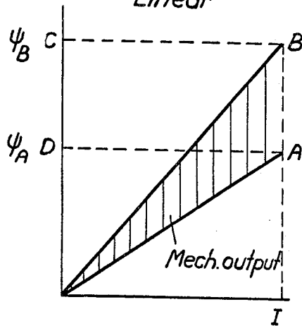
Fig. 9. Linear
