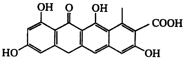
TETRACENOMYCIN F1 (5)
