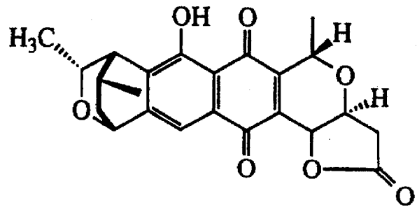
GRANATICIN (4)
