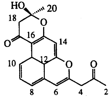
RM 20 (9)
