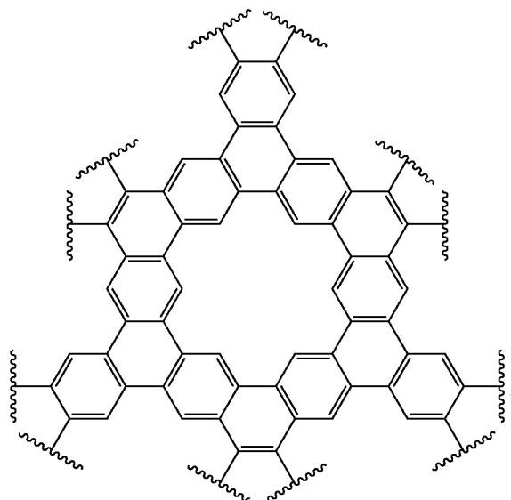
(XIX)
