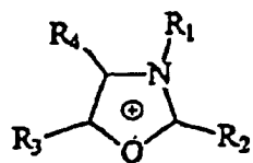
Oxazolium
