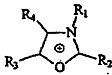
Oxazolium
