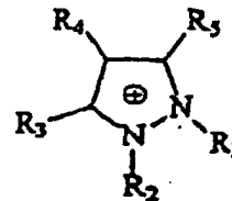
Pyrazolium
