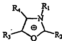
Oxazolium
