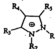
Pyrazolium
