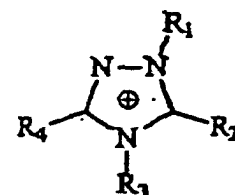
Triazolium
