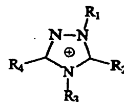
Triazolium
