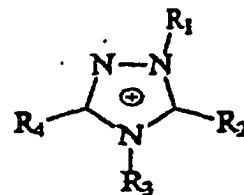
Triazolium
