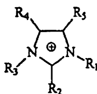
Imidazolium
