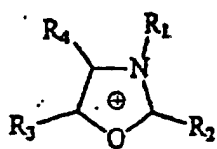
Oxazolium
