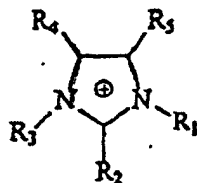
Imidazolium
