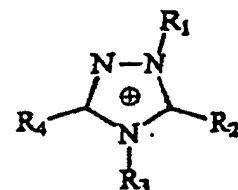
Triazolium
