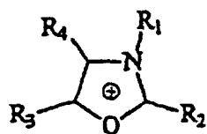
Oxazolium
