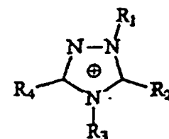
Triazolium
