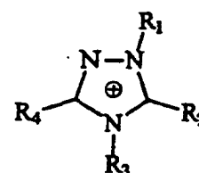
Triazolium
