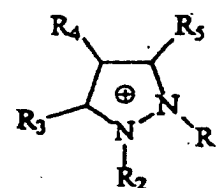
Pyrazolium
