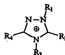
Triazolium
