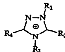
Triazolium
