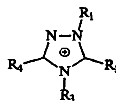
Triazolium
