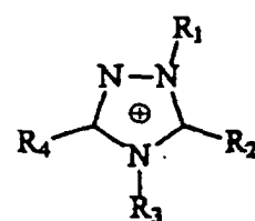
Triazolium
