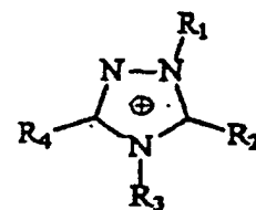
Triazolium
