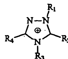
Triazolium
