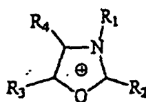
Oxazolium
