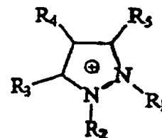
Pyrazolium
