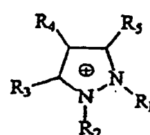
Pyrazolium
