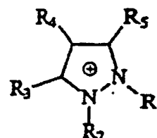
Pyrazolium
