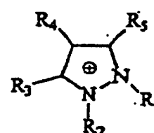
Pyrazolium
