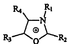
Oxazolium
