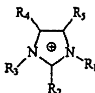
Imidazolium
