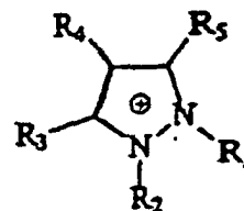
Pyrazolium
