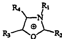
Oxazolium
