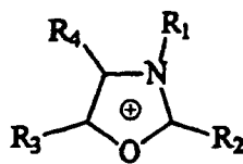
Oxazolium
