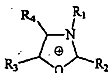
Oxazolium
