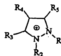
Pyrazolium
