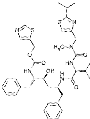
Ritonavir:
