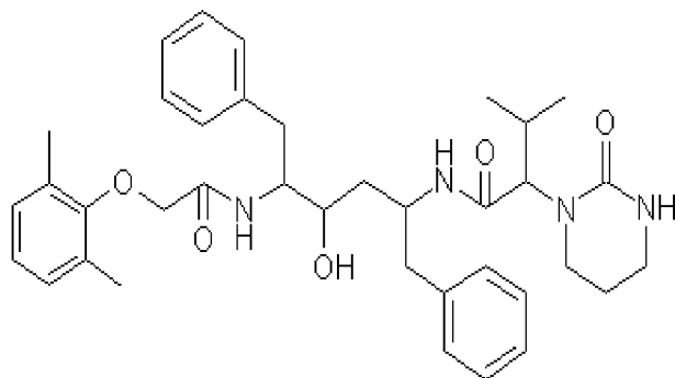
Ritonavir:
