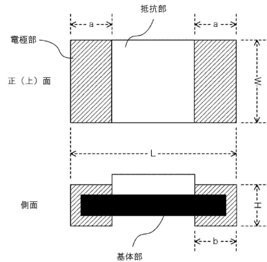
チップ抵抗 (10Ω~10MΩ) サイズ表
