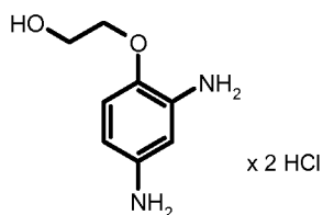
(VIa) molare Masse = 241,22 g/mol
