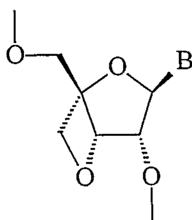
3'-4' D-form LNA
