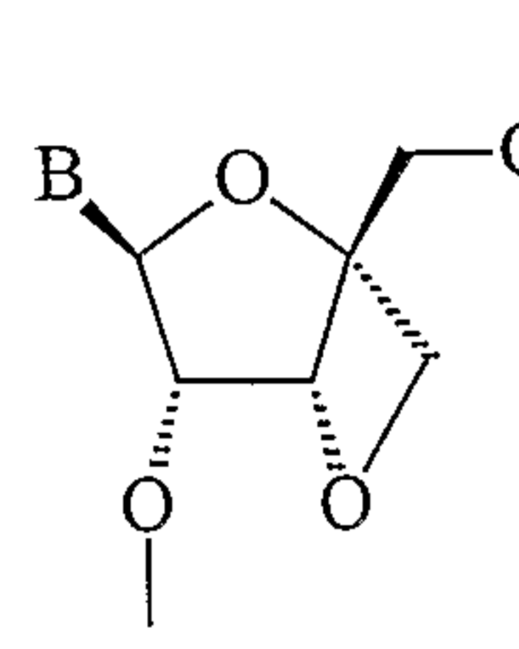
3'-4' L-form LNA
