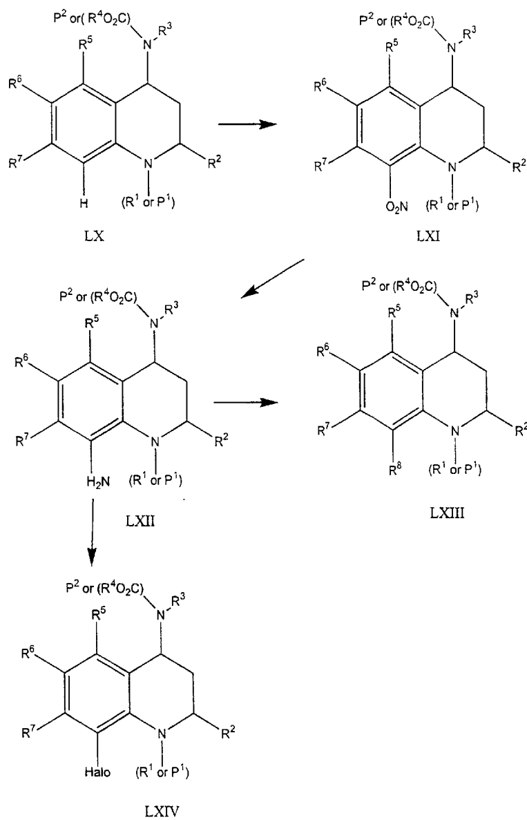
SCHEME VI
