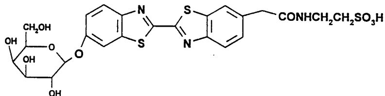
1m (BBTAATG):
