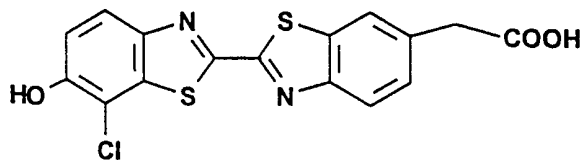
1h (ClBBTAA):
