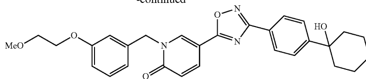
5-(3-(4-(1-Hydroxycyclohexyl)phenyl)-1,2,4-oxadiazol-5-yl)-1-(3-(2-methoxyethoxy)benzyl)pyridin-2(1H)-one
