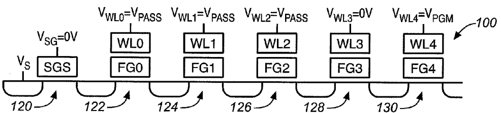
FIG. 6E (PRIOR ART)
