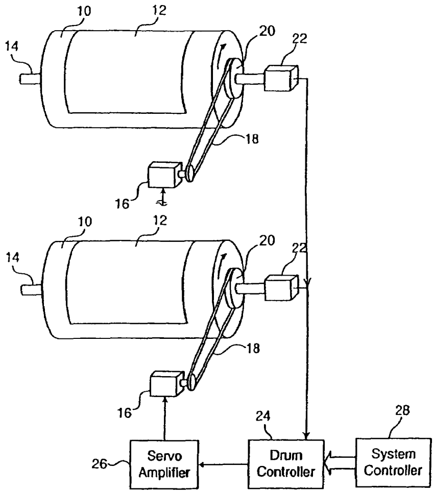
FIG. 1-A PRIOR ART
