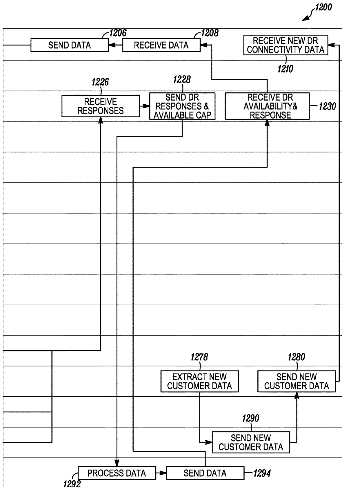
FIG. 12C
