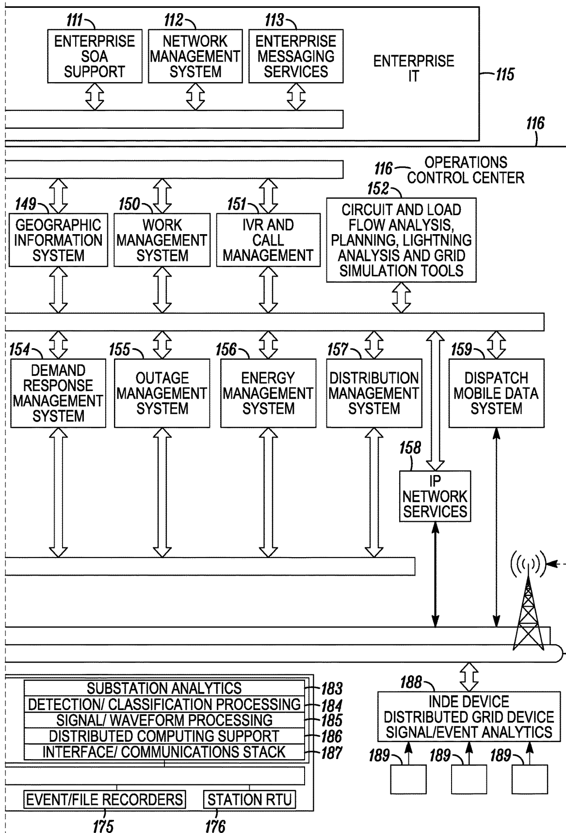
FIG. 3C
