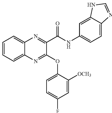
N-(1H-benzo[d]imidazol-6-yl)-3-(4-fluoro-2-methoxyphenoxy)quinoxaline-2-carboxamide
