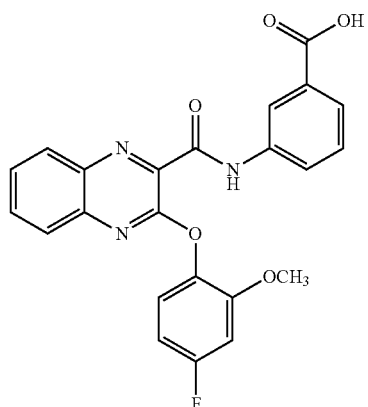
3-(3-(4-fluoro-2-methoxyphenoxy)quinoxaline-2-carboxamido)benzoic acid
