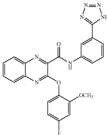
N-(3-(1H-tetrazol-5-yl)phenyl)-3-(4-fluoro-2-methoxyphenoxy)quinoxaline-2-carboxamide
