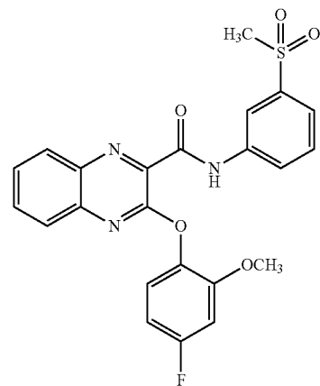
3-(4-fluoro-2-methoxyphenoxy)-N-(3-(methylsulfonyl)phenyl)quinoxaline-2-carboxamide
