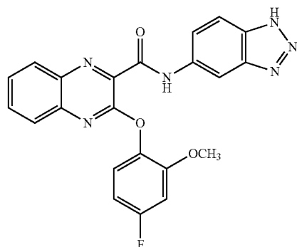
N-(1H-benzo[d][1,2,3]triazol-5-yl)-3-(4-fluoro-2-methoxyphenoxy)quinoxaline-2-carboxamide
