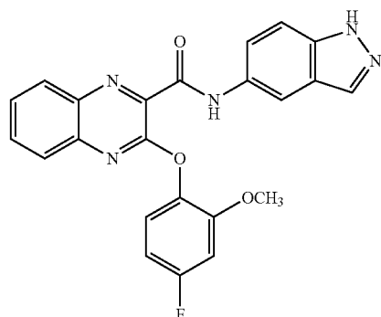
3-(4-fluoro-2-methoxyphenoxy)-N-(1H-indazol-5-yl)quinoxaline-2-carboxamide
