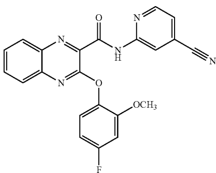
N-(4-cyanopyridin-2-yl)-3-(4-fluoro-2-methoxyphenoxy)quinoxaline-2-carboxamide
