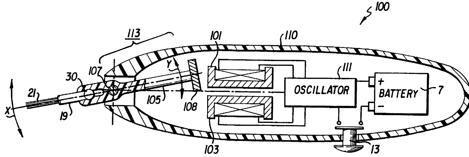
FIG. 9
