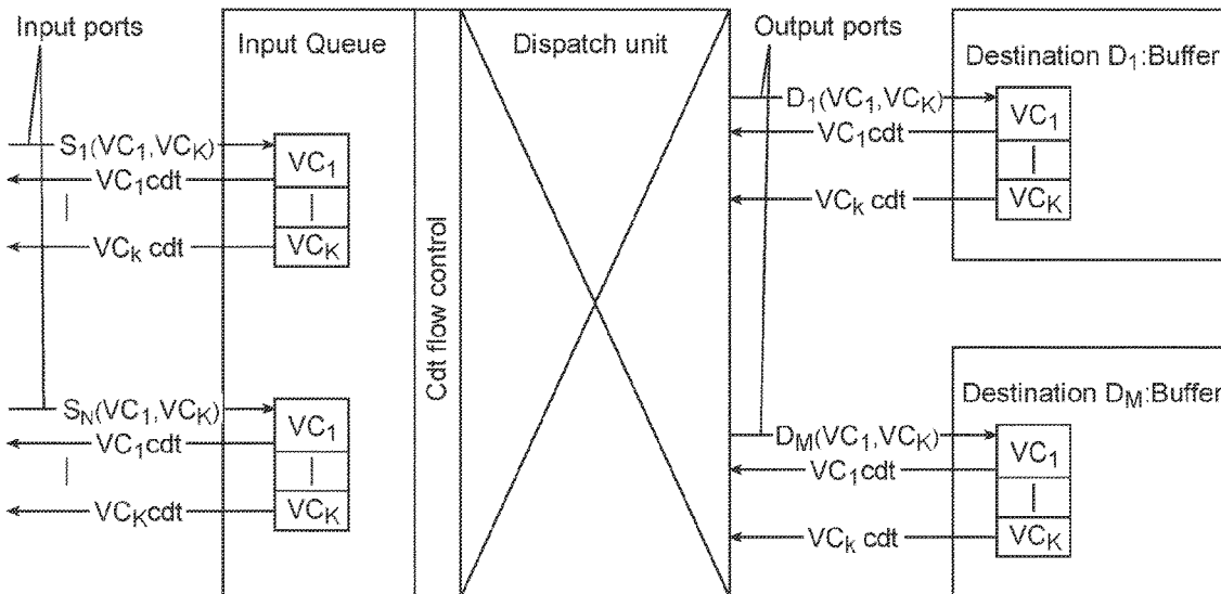
Input Queue switch
