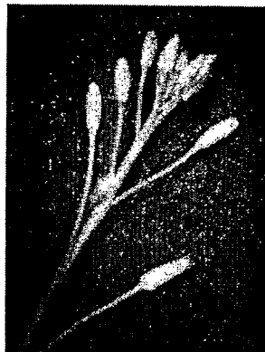
35S::MNT RNAi line 3
