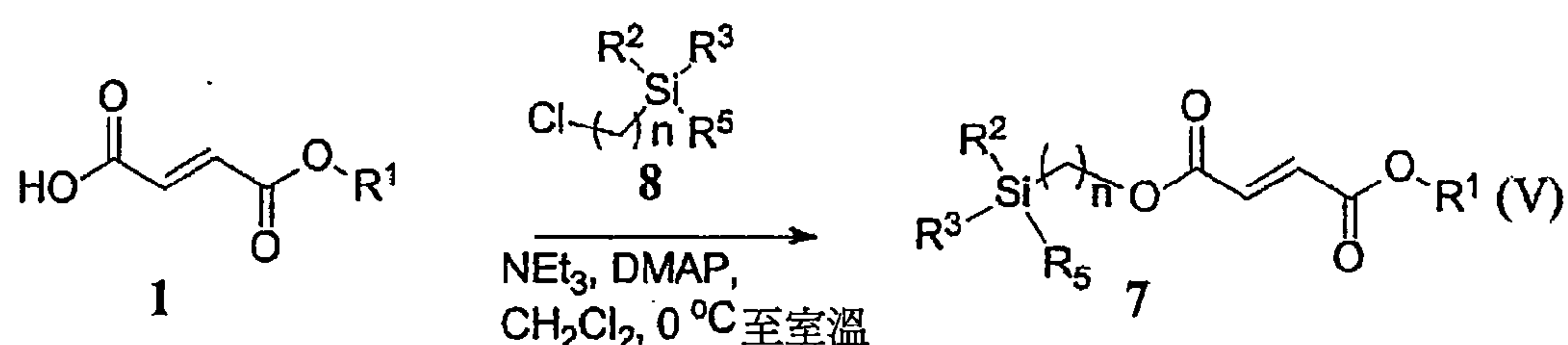
反應圖 8
