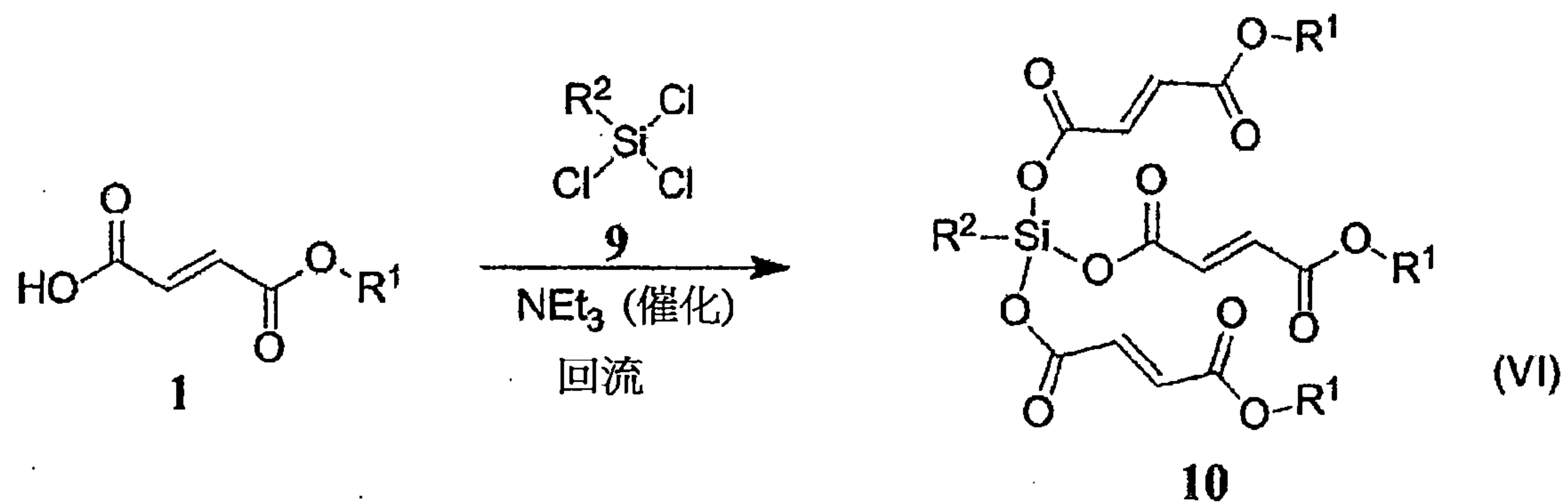
反應圖 9
