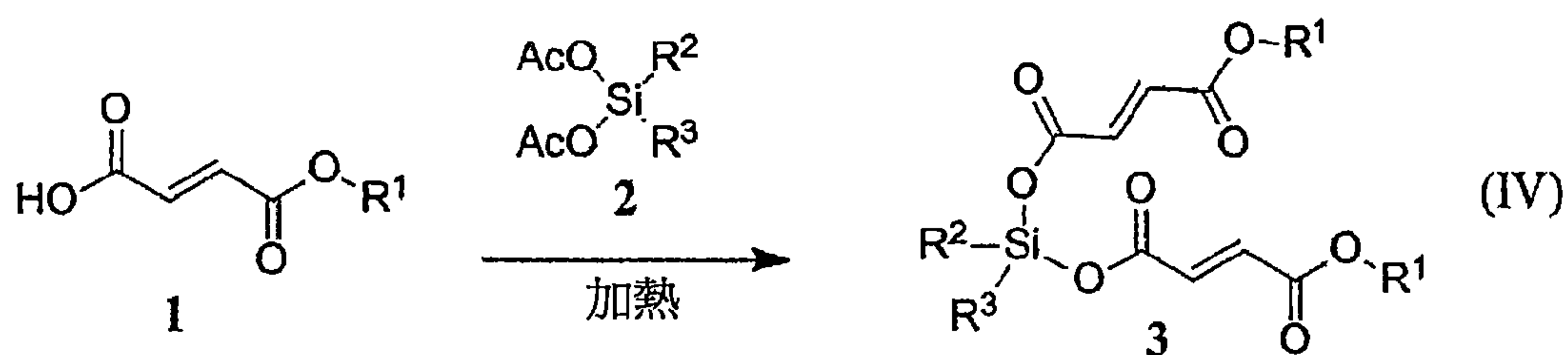
反應圖 1
