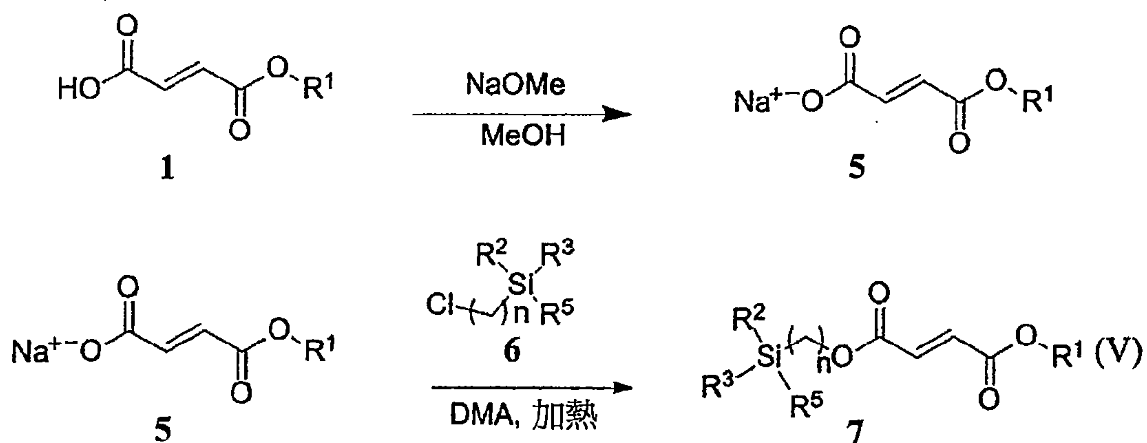
反應圖 6
