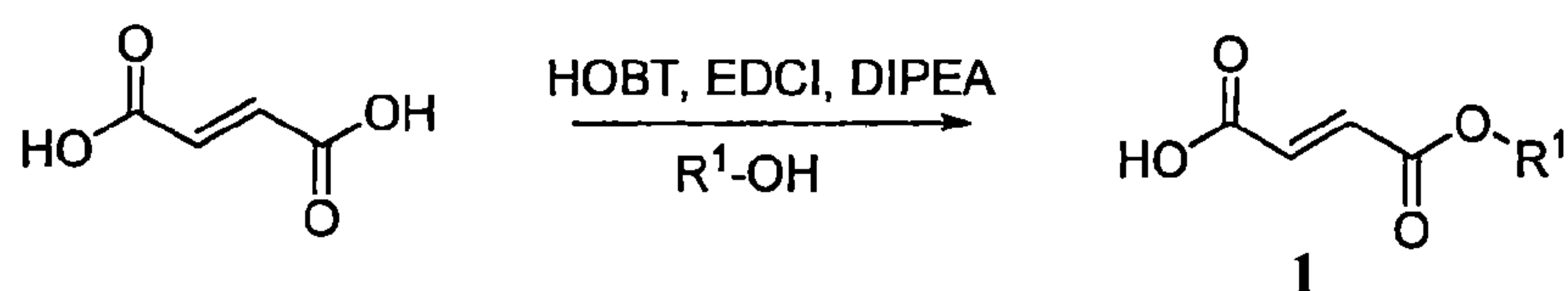
反應圖 3
