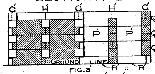
FIG. 3' SECTION C-D
