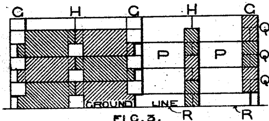
FIG. 3. SECTION C-D
