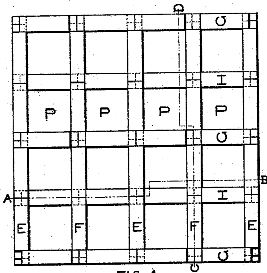
FIG. 1 PLAN
