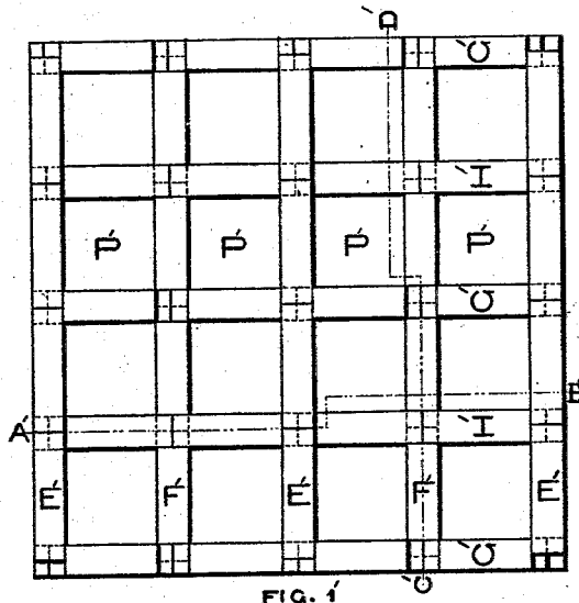
FIG. 1' PLAN
