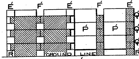
FIG. 2' SECTION A-B
