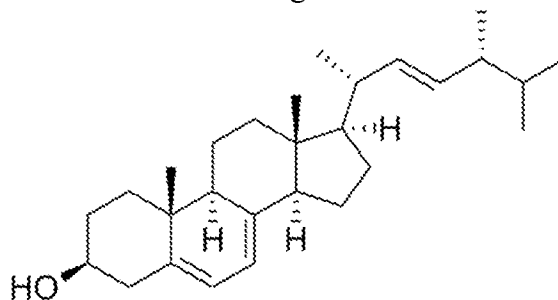
Ergosterol
