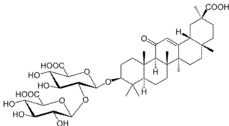
Glycyrrhizic acid
