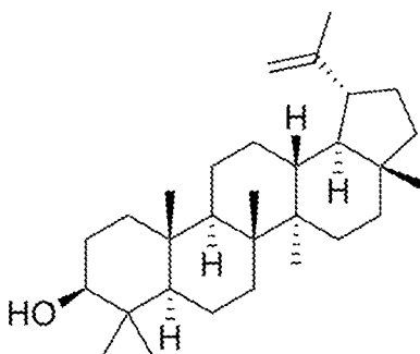
Lupeol
