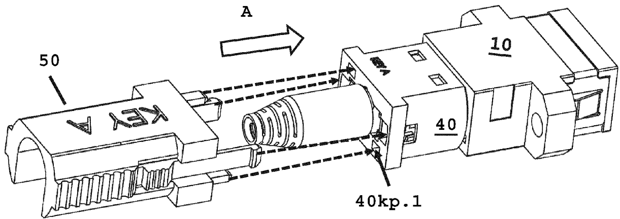
FIG. 13A
