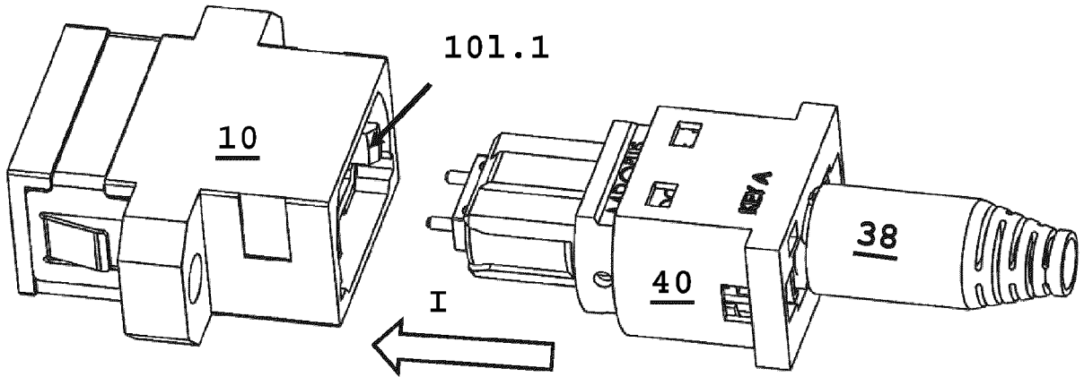
FIG. 10A
