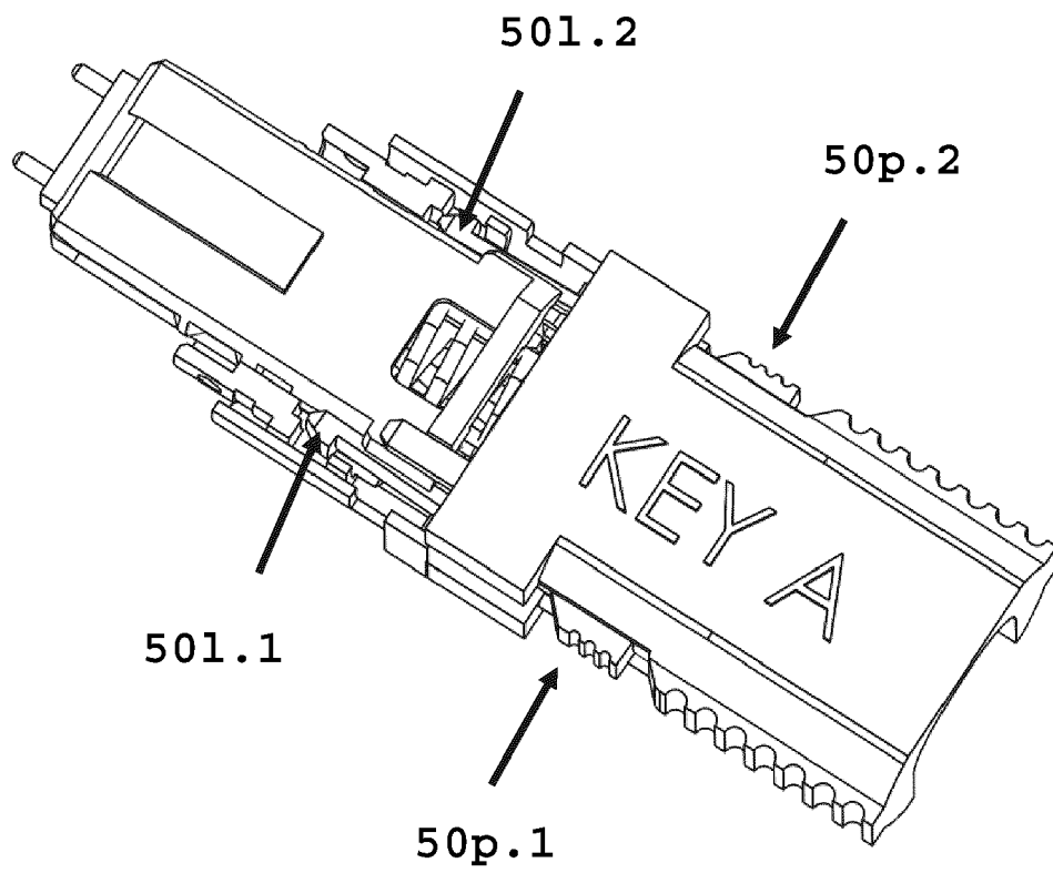
FIG. 14D
