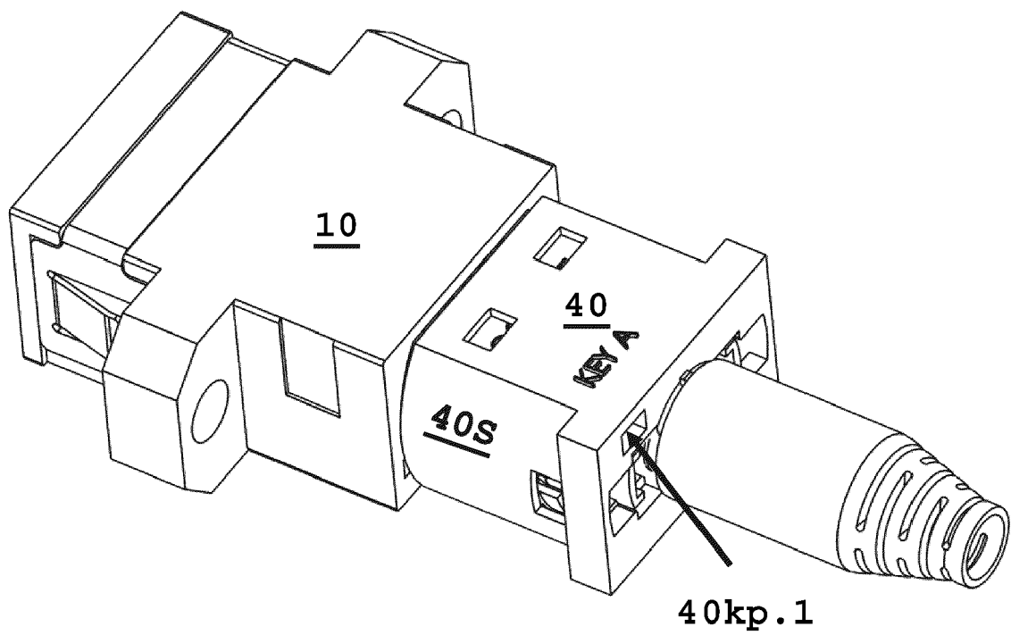
FIG. 10E
