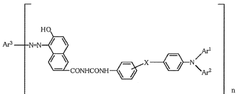
Allgemeine Formel (2)
