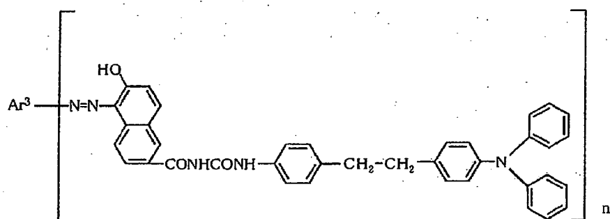
Formule générale (3)
