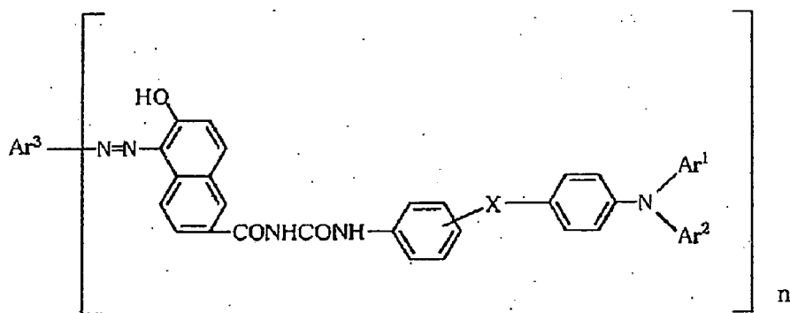
Formule générale (2)
