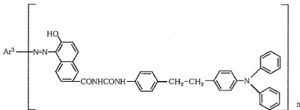
Allgemeine Formel (3)
