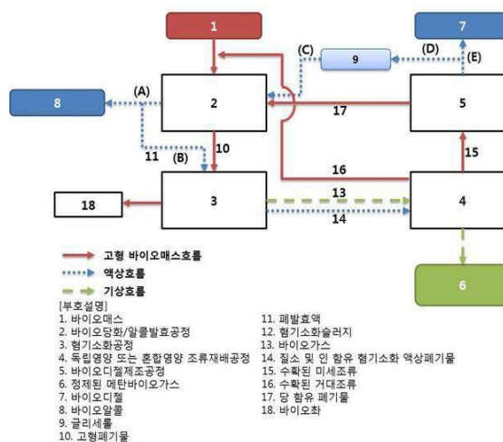
Waste Zero 바이오에너지 생산공정
