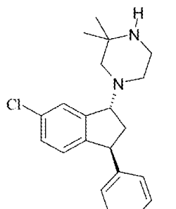
(XI)
