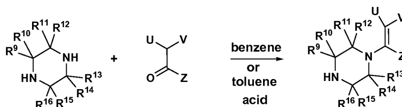
Scheme VI
